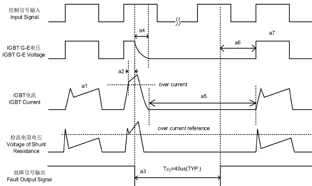
图 6.过流保护
