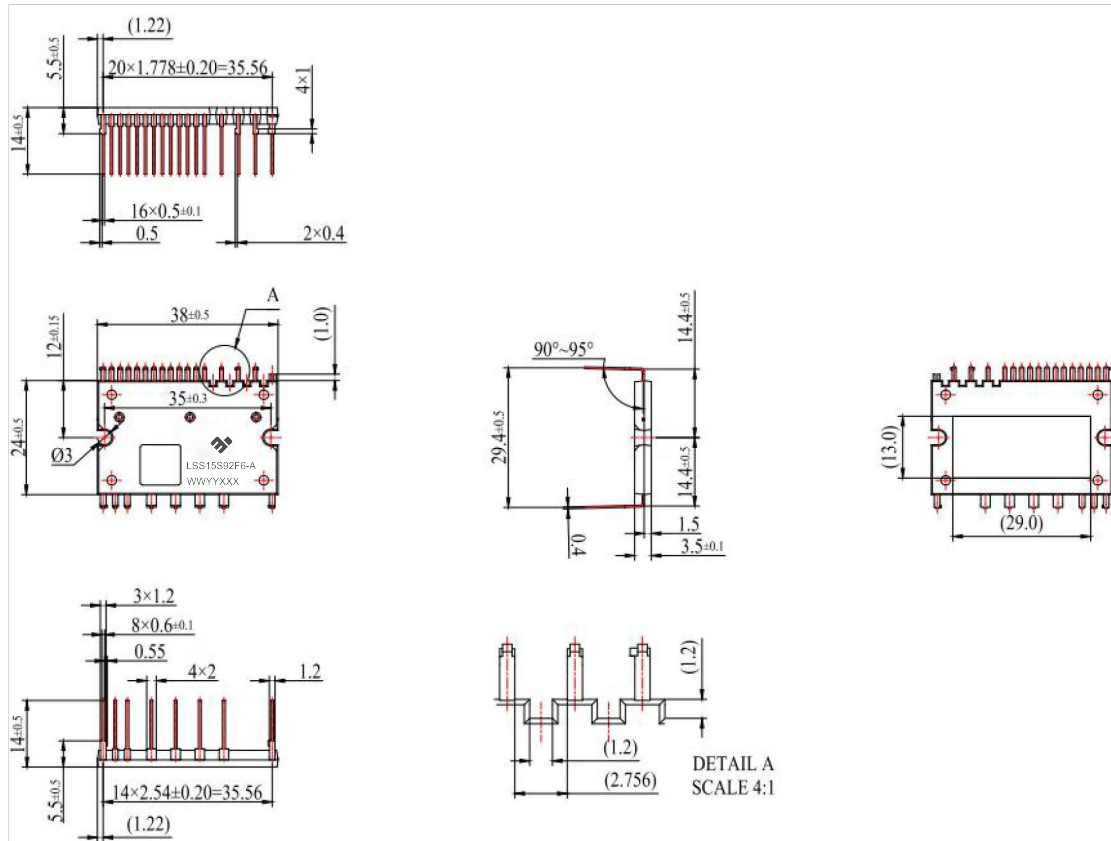
图 9. 封装轮廓详图 Fig 9. Detailed Package Outline Drawings
