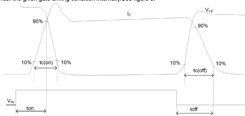
图 3.开关时间定义 Fig 3. Switching Time Definition
