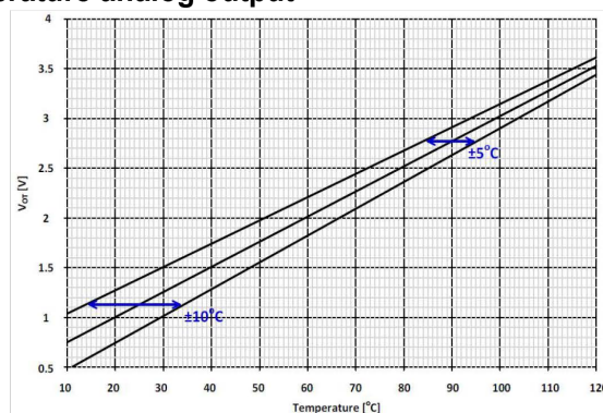
图 4. 温度输出电压
