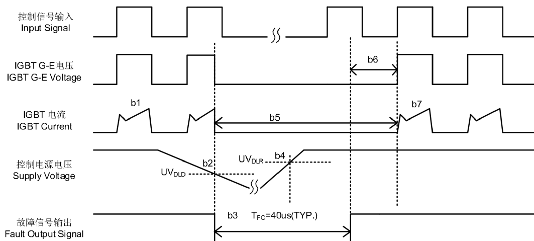
图 7.下桥欠压保护
