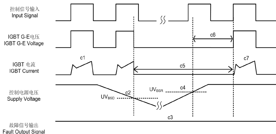
图 8.上桥欠压保护
