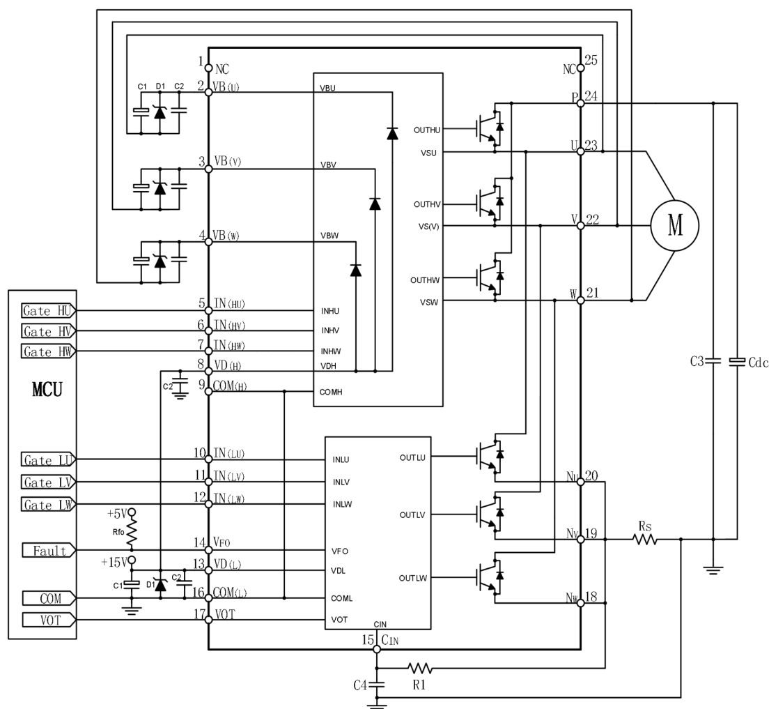
图 9. 典型应用电路 Fig 9. Typical Application Circuit
