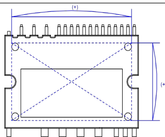
图 5. 平面度测量位置 Fig 5. Flatness Measurement Position
